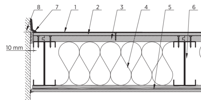
Rys. 7. Detal wykończenia podkładu podłogowego wzdłuż ściany (Opis: 1. Warstwy wykończeniowe podłogi, 2. Płyty HYDROPANEL/CEMENTEX, 3. Płyty DURIPANEL, 4. Materiał izolacyjny, 5. Zabudowa sufitowa, 6. Nośna konstrukcja stalowa C254, 7. Listwa podłogowa, 8. Ściana)
