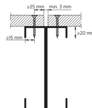
Rys 1. Schemat mocowania płyt DURIPANEL za pomocą wkrętów
