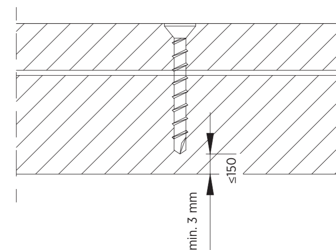
Rys 5. Schemat mocowania płyt HYDROPANEL/CEMENTEX
