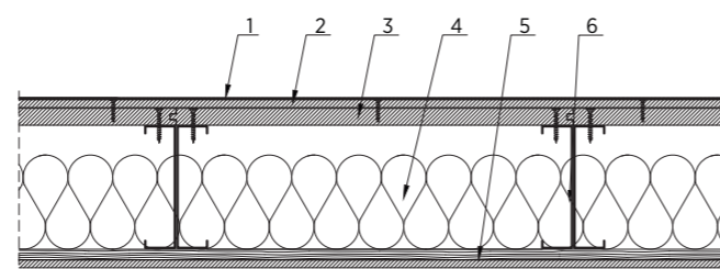
Rys. 1. Strop stalowy z zabudową sufitową zamocowaną bezpośrednio do spodu stropu (Opis: 1. Warstwy wykończeniowe podłogi, 2. Płyty HYDROPANEL/CEMENTEX, 3. Płyty DURIPANEL, 4. Materiał izolacyjny, 5. Zabudowa sufitowa, 6. Nośne profile stalowe).
